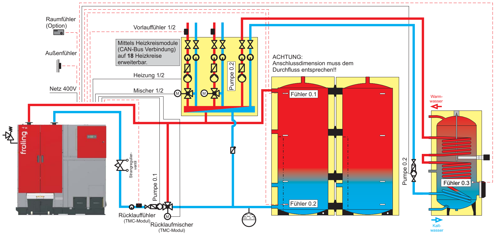
Hackgutfeuerung TX 150
